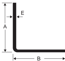
ÁNGULOS DE ACERO INOXIDABLE STAINLESS STEEL ANGLES ANGLES EN ACIER INOXYDABLE
