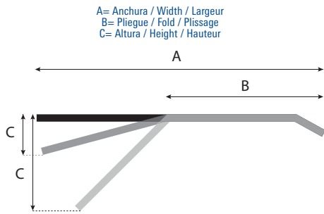
DIFERENCIA DE NIVEL DE ACERO ST. STEEL LEVEL DIFFERENCE DIFFÉRENCE DE NIVEAU ACIER
